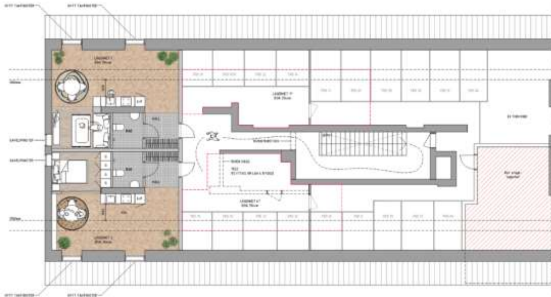
Planlösning med 2st smålägenheter som exempel
